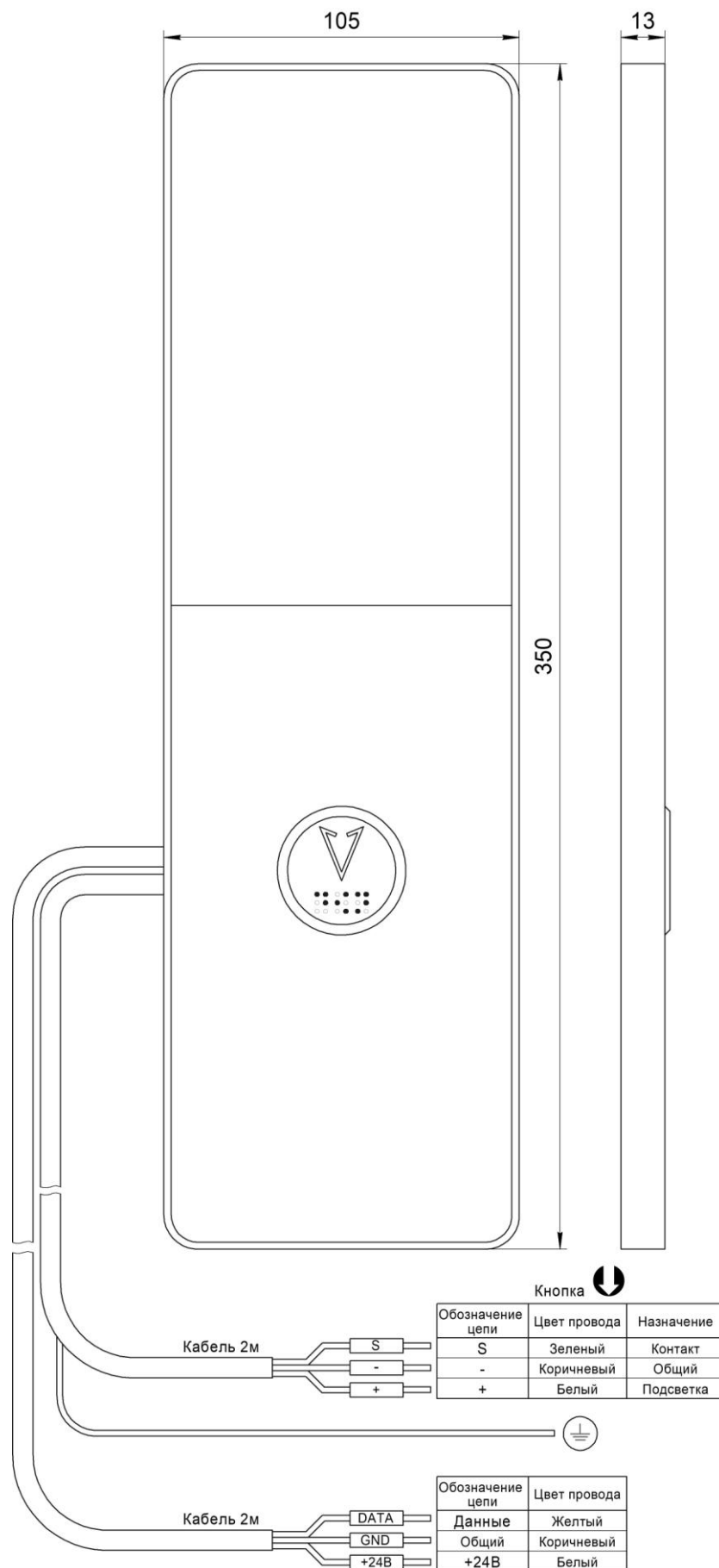
Рис.1 Внешний вид, габаритные и установочные размеры Вызывного поста МАЛАХИТ НШЕК.468381.025-01
